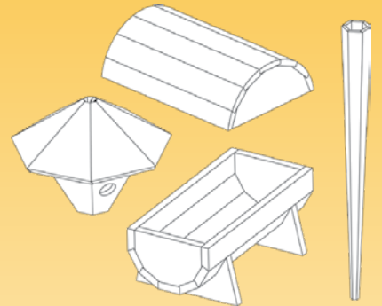
Noen eksempler på ting man kan lage med disse fresestålene.
